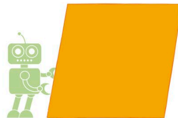
Rhombus
