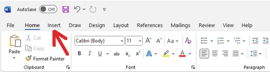
Fig. 14.1 Insert button
